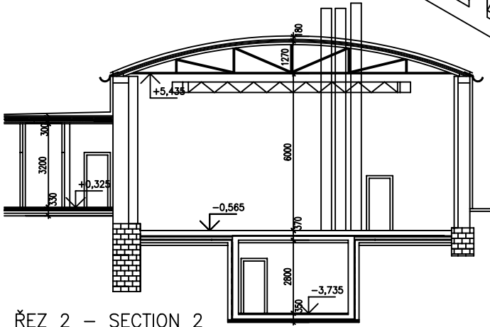
ŘEZ 2 – SECTION 2
